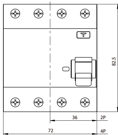
TYB2L-100
