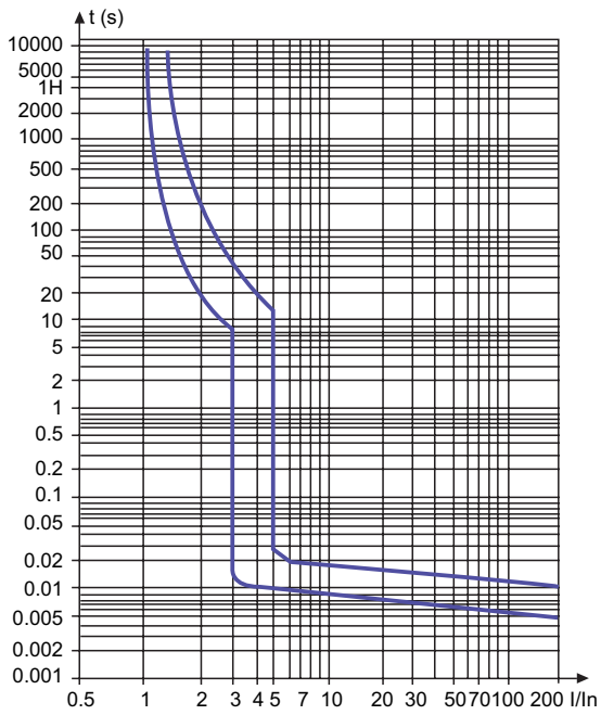
B 曲线
