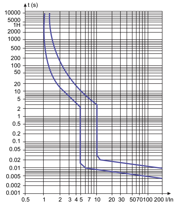
C 曲线
